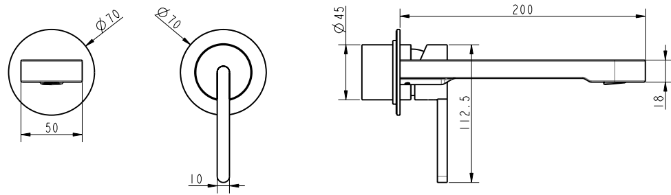
ברז קיר נסתר קומפלט BM5236
