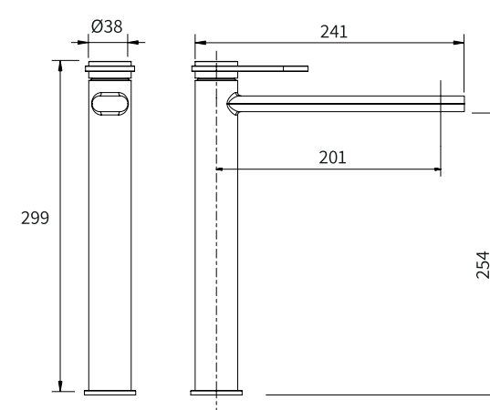
ברז פרח קבוע נמוך BM5320
