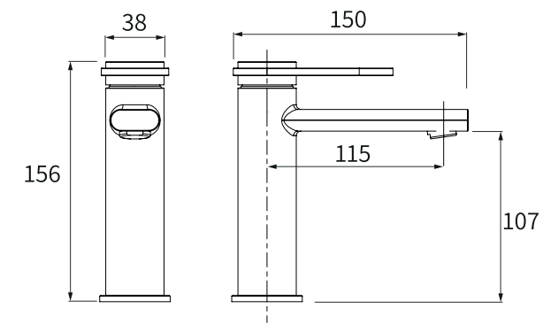
BM5157 ברז פרח קבוע נמוך
