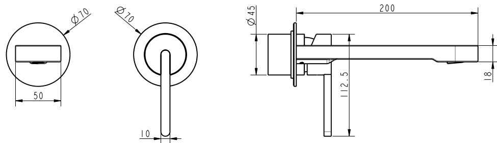
ברז קיר נסתר קומפלט BM5294
