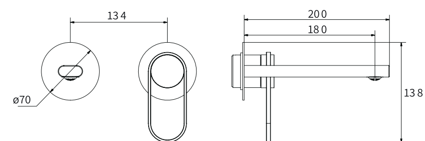
BM5153 ברז פרח קבוע גבוה
